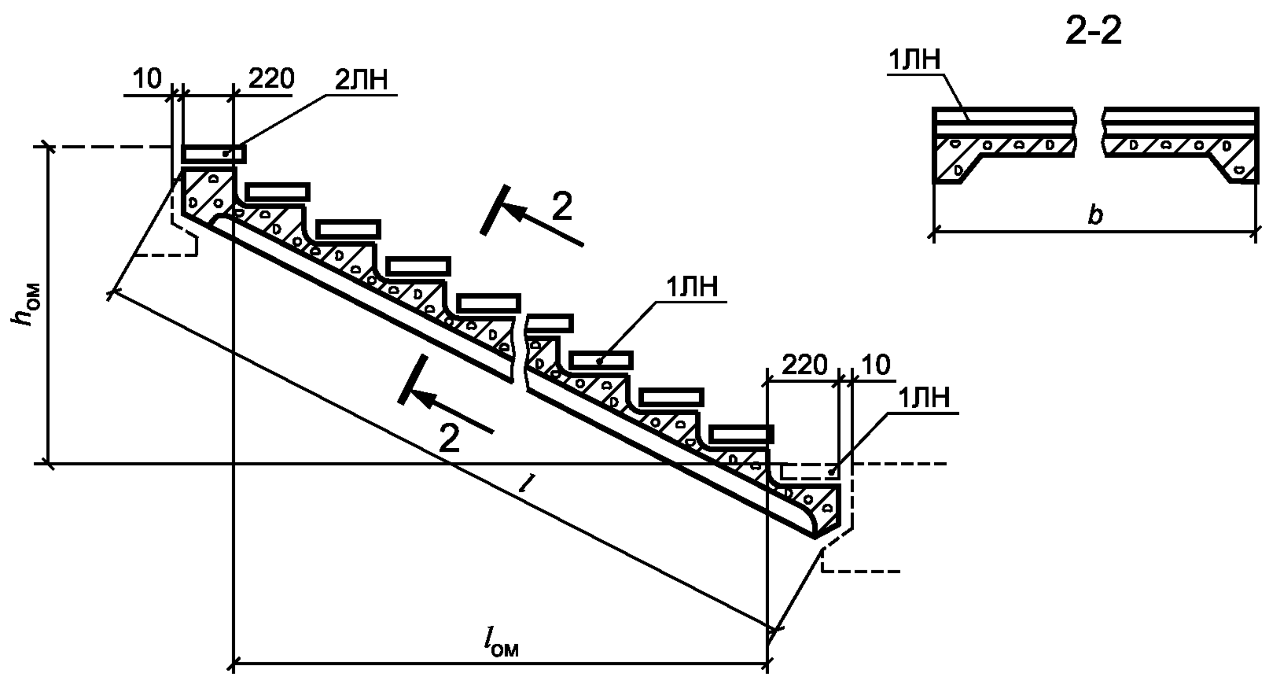
Рисунок 2 — Марш типа ЛМФ
