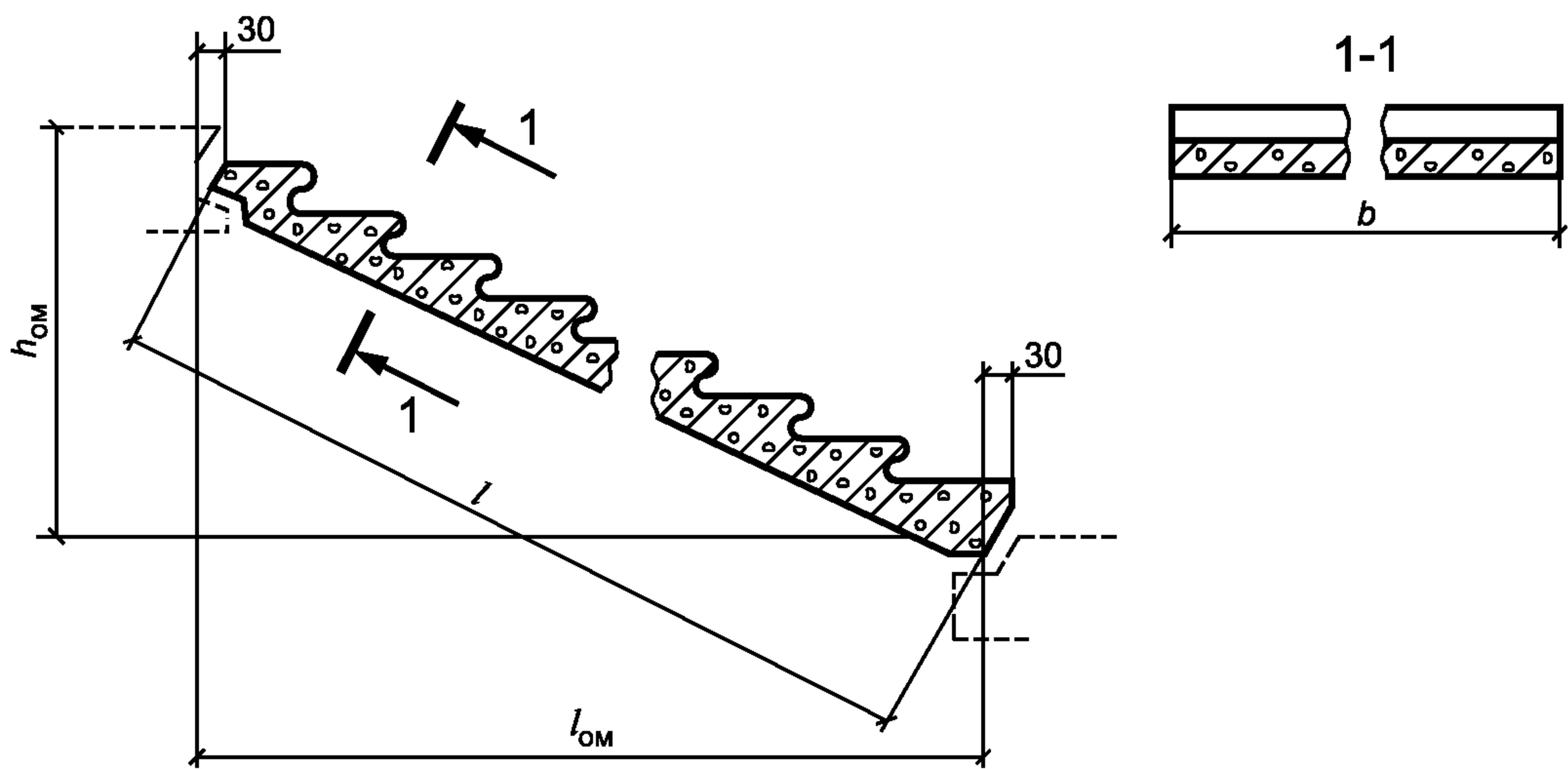
Рисунок 1 — Марш типа ЛМ
